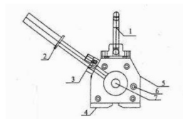
Сборочные детали магнитного захвата
