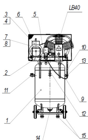
Общий вид компрессора СБ4/С-100.LB40В
