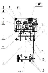
Общий вид компрессора СБ4/С-100.LB40В
