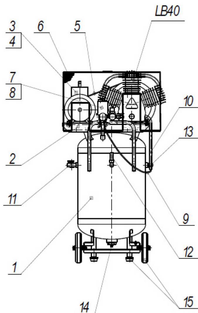
Общий вид компрессора СБ4/С-100.LB40B
