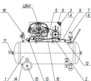
Общий вид компрессора СБ4/С-200.LB40
