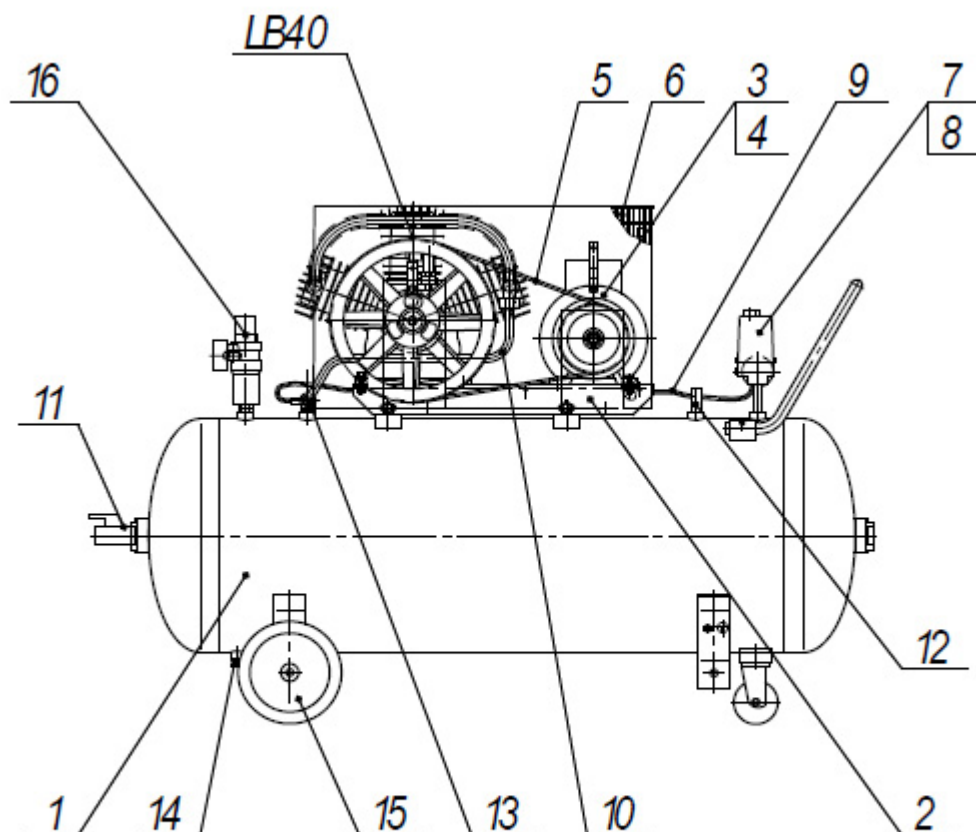
Общий вид компрессора СБ4/С-200.LB40
