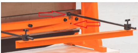
Регулируемый ограничитель подачи листа – 550мм
