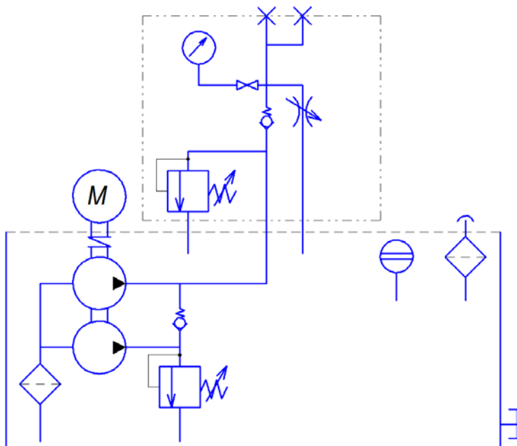
Рис.2 (Гидравлическая схема)
