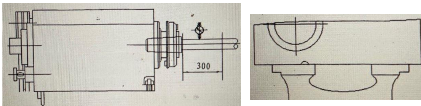
Рис.6 - Регулировка точности напорного ящика
