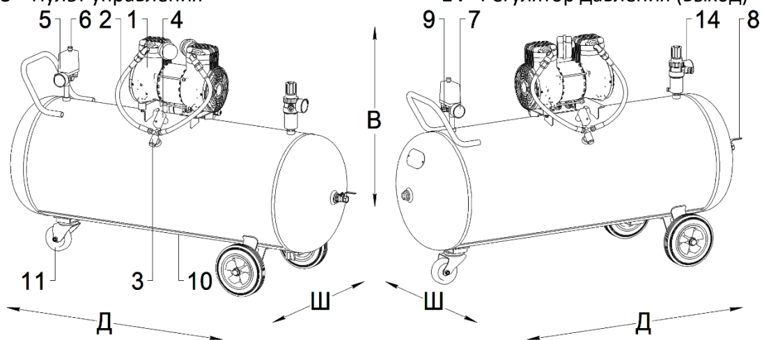
Рисунок 9 - Общий вид компрессора СБ4/С-200.OLD30(А)
