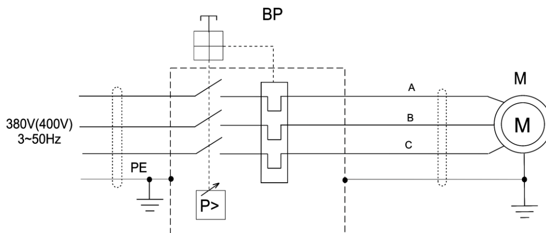
Рисунок А.1 - Схема электрическая принципиальная компрессора СБ4/С-50.OLD30А, СБ4/С-100.OLD30А
