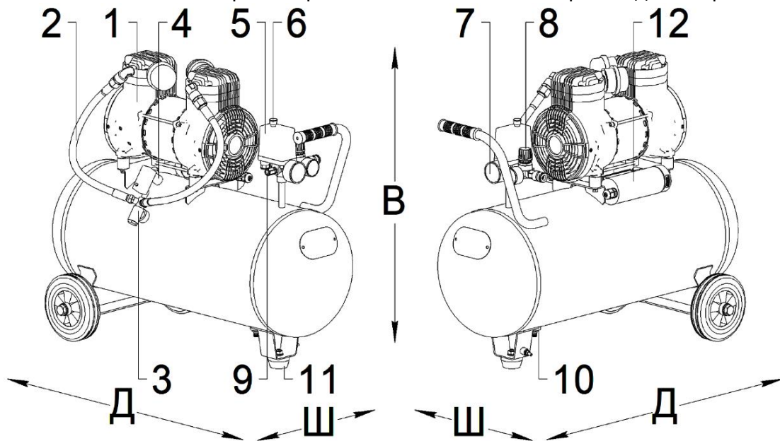
Рисунок 7 - Общий вид компрессора СБ4/С-50.OLD30(А)
