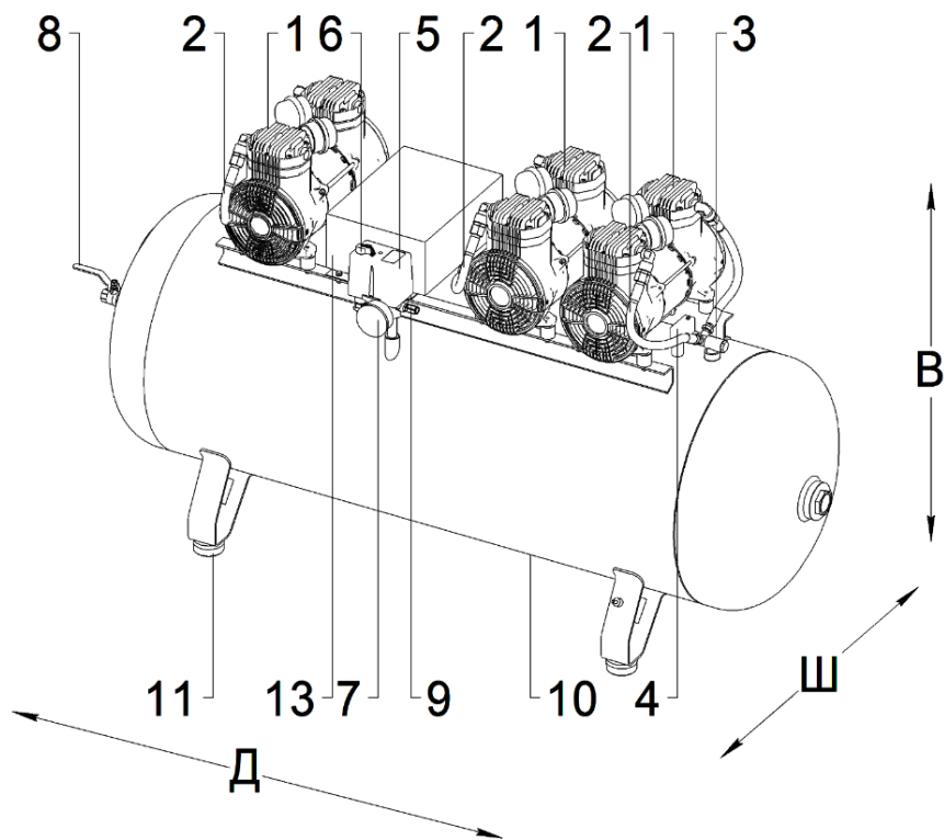
Рисунок 11 - Общий вид компрессора СБ4/Ф-270.OLD30Т
