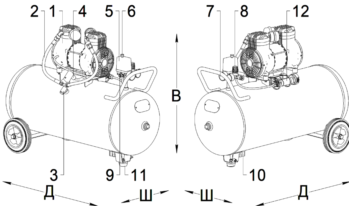
Рисунок 8 - Общий вид компрессора СБ4/С-100.OLD30(А)
