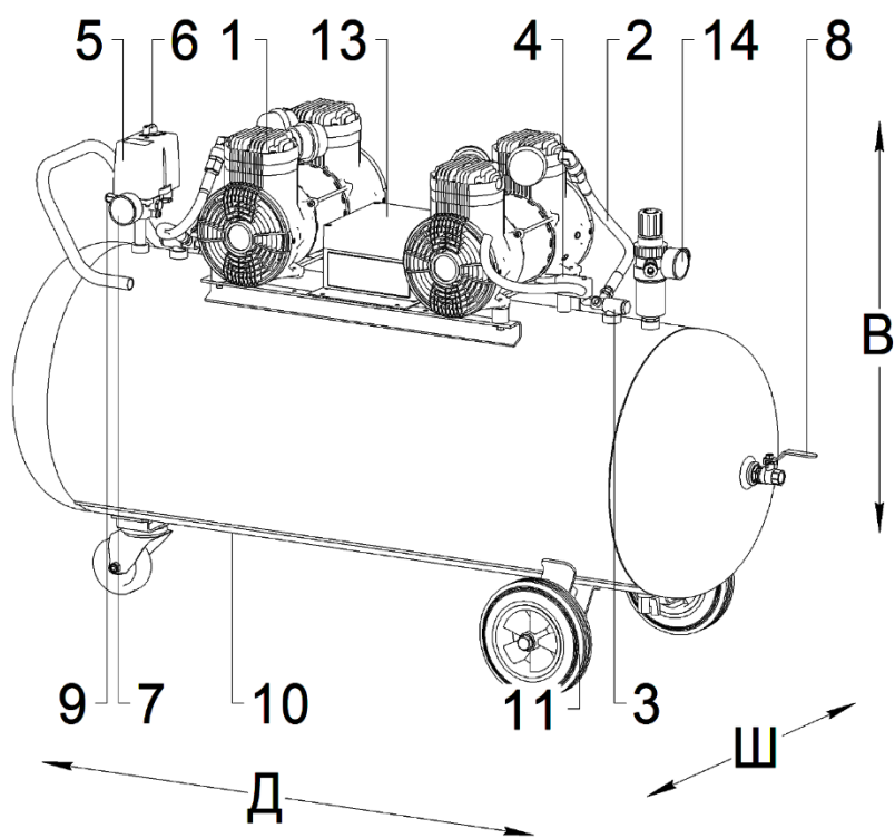
Рисунок 10 - Общий вид компрессора СБ4/С-200.OLD30Т
