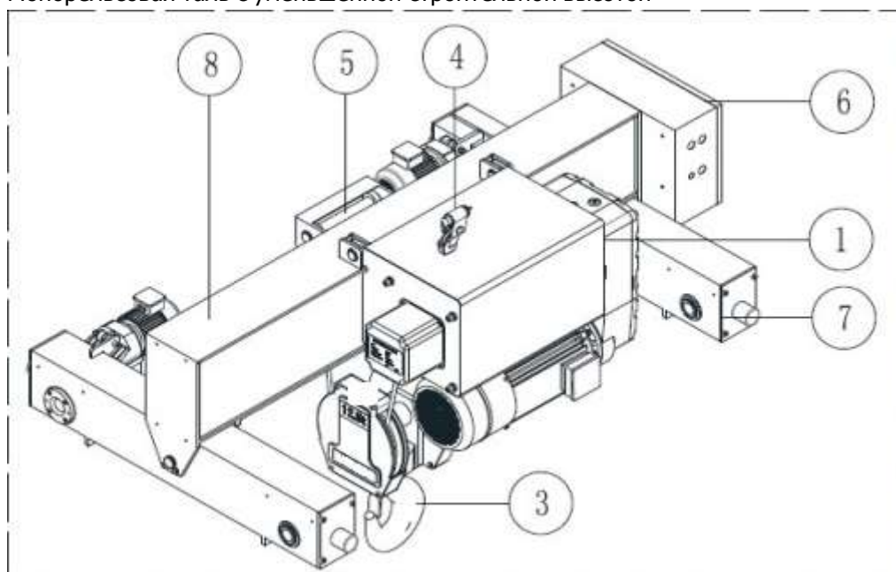
Монорельсовая таль с уменьшенной строительной высотой
