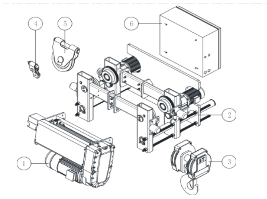
Монорельсовая таль с уменьшенной строительной высотой
