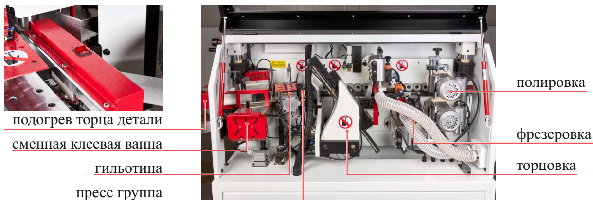
Устройство кромкооблицовочной линии. Рис. №2
