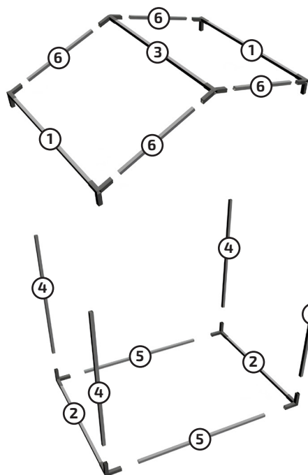
Рис. 2. Схема сборки каркаса палатки сварщика.
