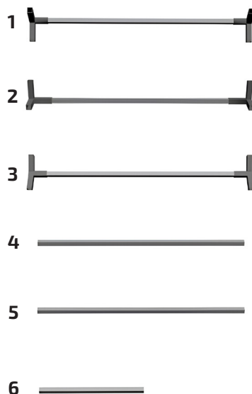
Рис. 2. Схема сборки каркаса палатки сварщика.
