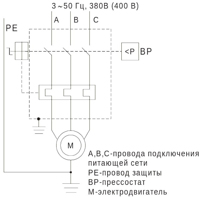
Рисунок А.1 - Схема электрическая принципиальная
